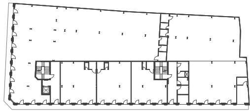
PLANTA BAJA
