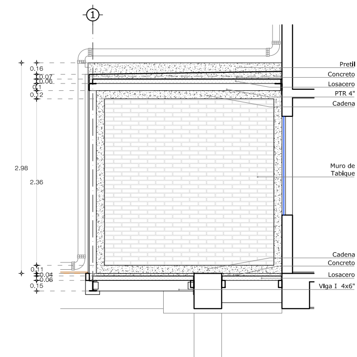
CORTE "B" / CONSTRUCTIVO
