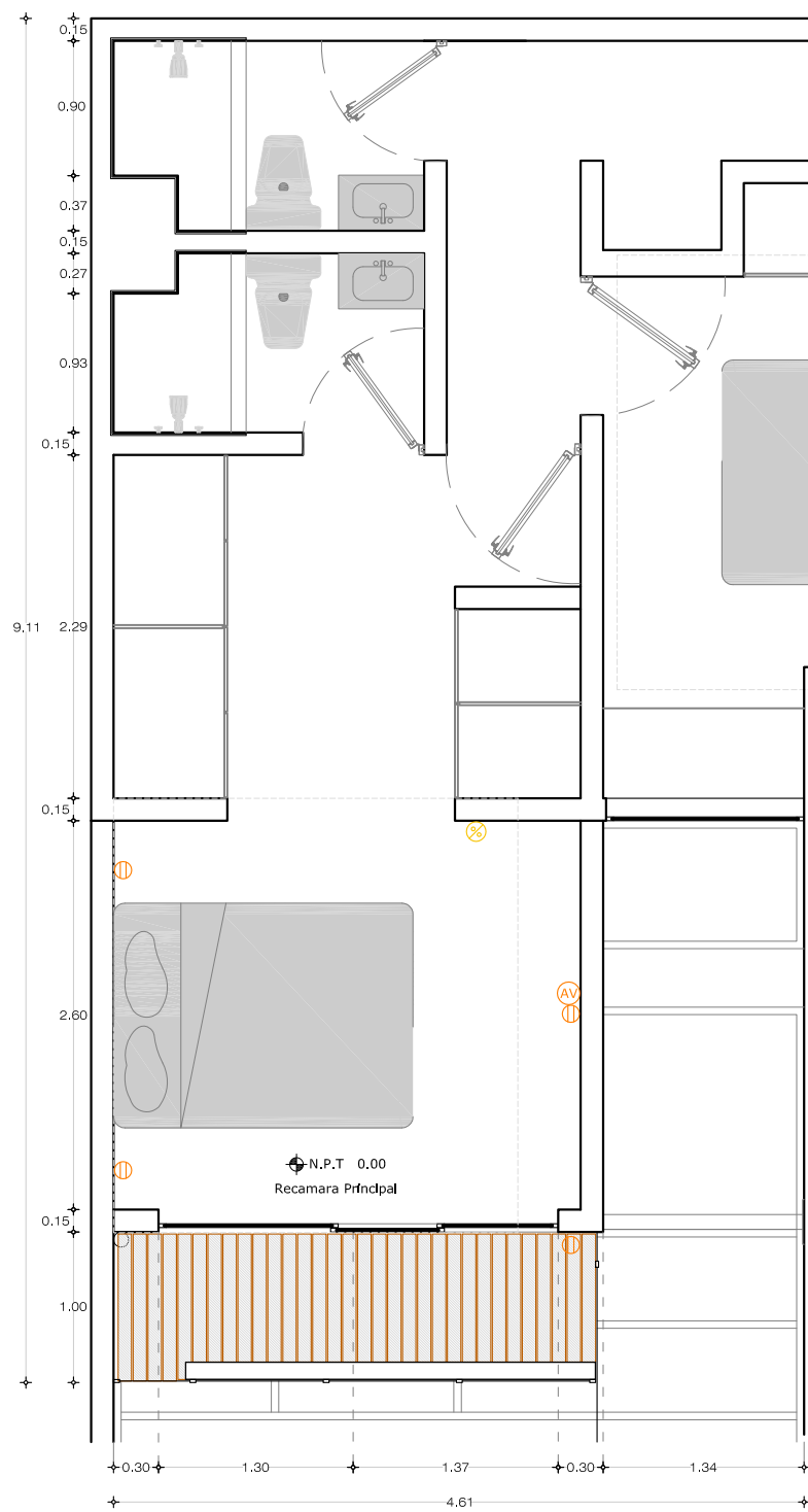
PLANTA ARQUITECTÓNICA
