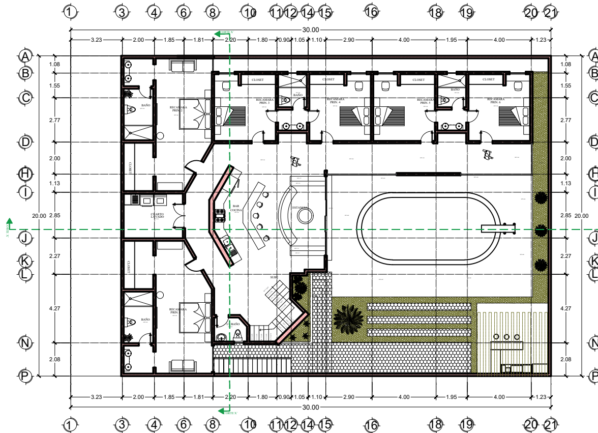
PLANTA BAJA PRIMER ETAPA
