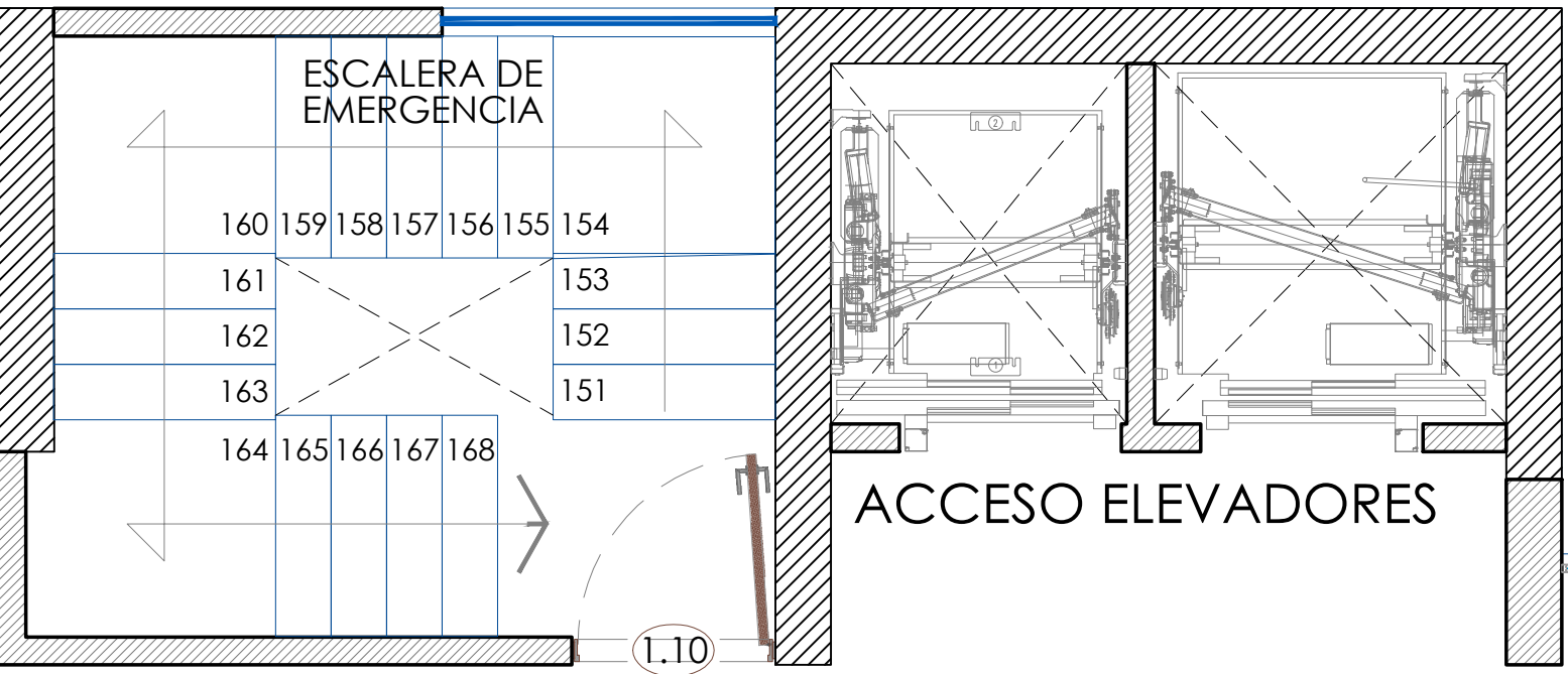
ÁREA COMÚN SIN VACIOS 81.59M²
