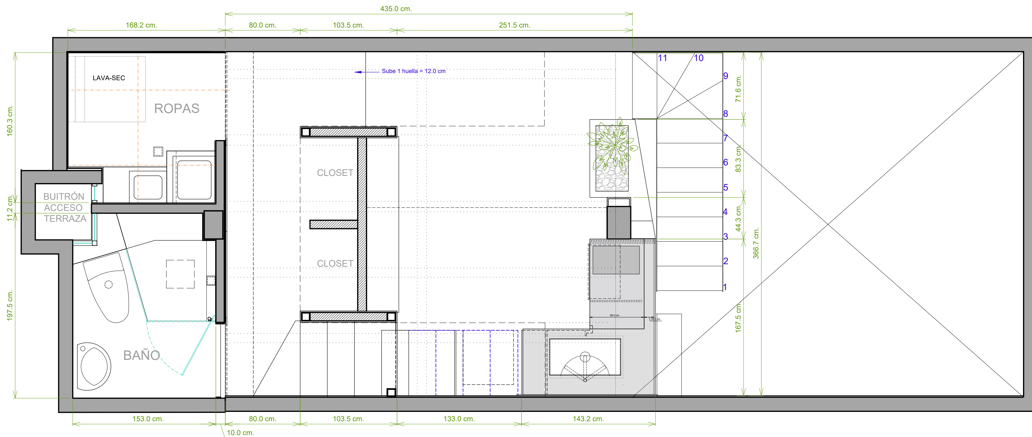
PLANTA PISO 2
